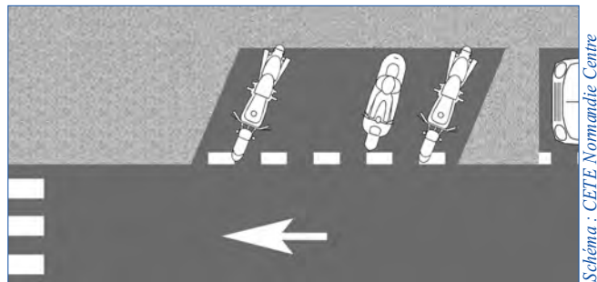
En épis (profondeur de l'encoche 2,00 m).
