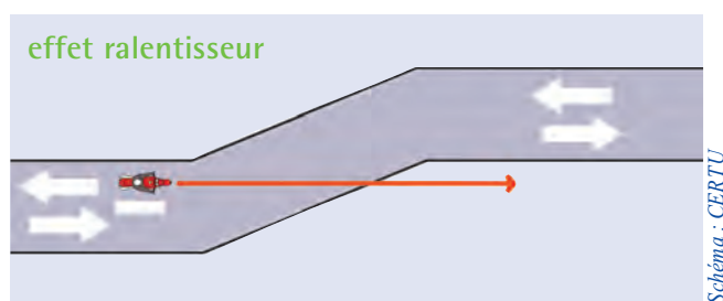
Illustration d'un aménagement présentant un déport géométrique égal à la largeur de voie, le deux-roues motorisé est ainsi obligé de modifier sa trajectoire.
