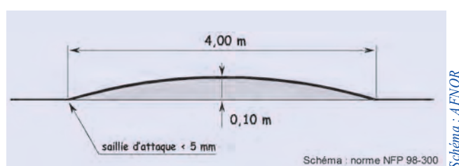
Ralentisseur de type dos-d'âne
